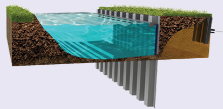
Keerwand grond en waterkering
