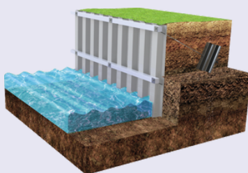
Kade toepassing
